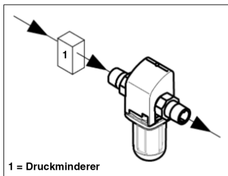
Abb. 2: Druckminderer vor dem Kerzenfilter
