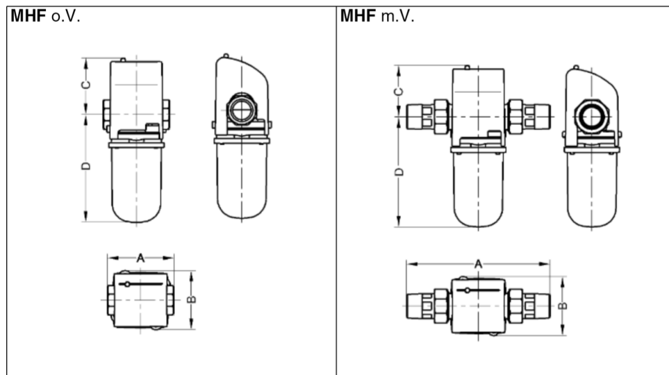
Abb. 1: Einbaumaße MHF
