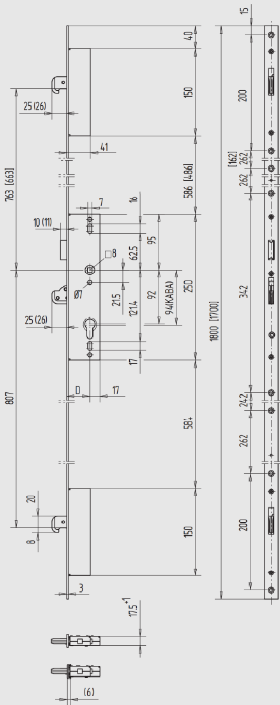
Abbildung DIN rechts (...) = U-Stulp [...] = Länge 1700 mm
