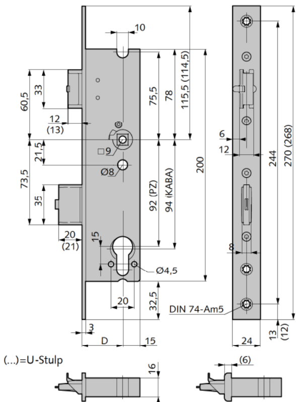
Abbildung zeigt Schloss mit geteilter Nuss, 2-flügelig
