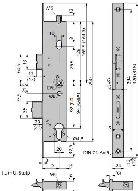
Abbildung zeigt Schloss mit oberer Zusatzverriegelung (ZV) und geteilter Nuss, 2-flügelig
