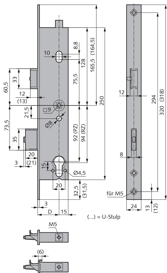
Abbildung zeigt Schloss mit oberer Zusatzverriegelung (ZV) und geteilter Nuss, 2-flügelig
