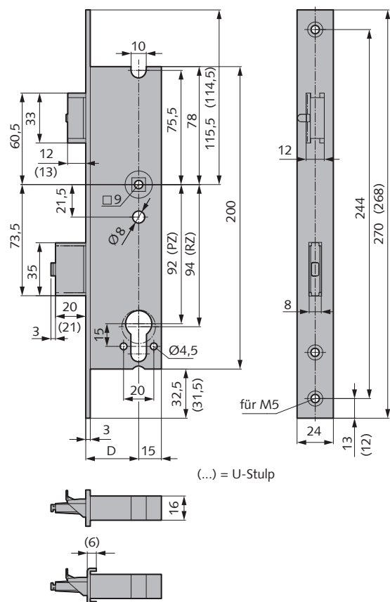
Abbildung zeigt Schloss mit geteilter Nuss, 2-flügelig
