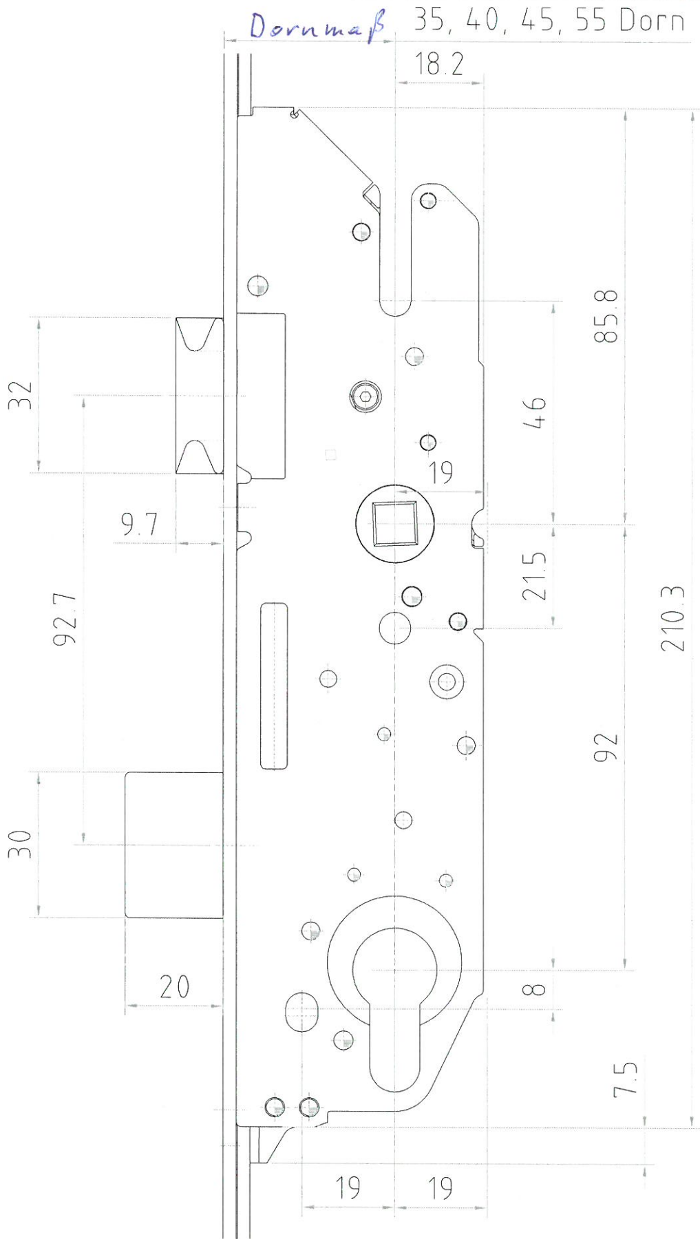
Schüring Schloßkasten für gleichläufige Riegeltechnik.
