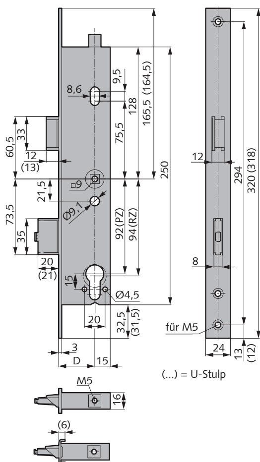
Abbildung zeigt Schloss mit geteilter Nuss und oberer Zusatzverriegelung (ZV), 2-flügelig
